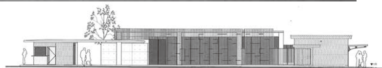
▲ PLAZA KIT 西立面図
